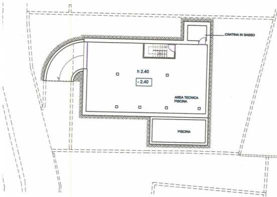
PIANTA PIANO INTERRATO - scala 1:200
