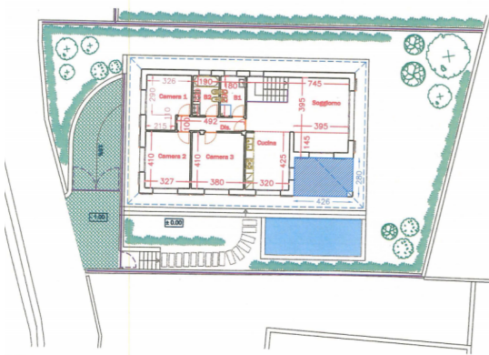
PIANTA PIANO TERRA - scala 1:200
